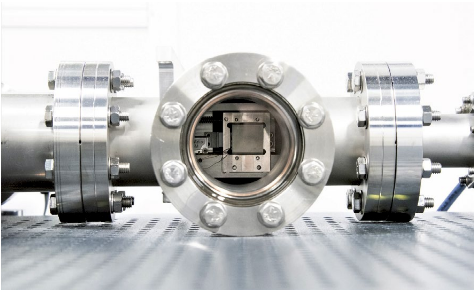
Test opstelling van KNUT motor in een Ultra Hoog Vacuüm kamer.
